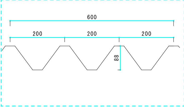
ルーフデッキH88折板
