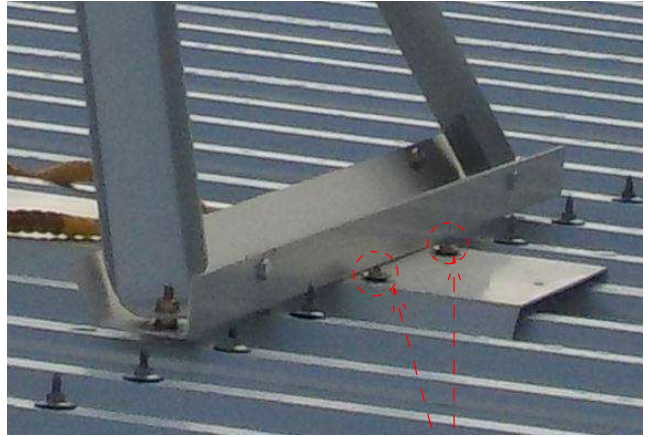
折板タイトフレームボルトに固定
