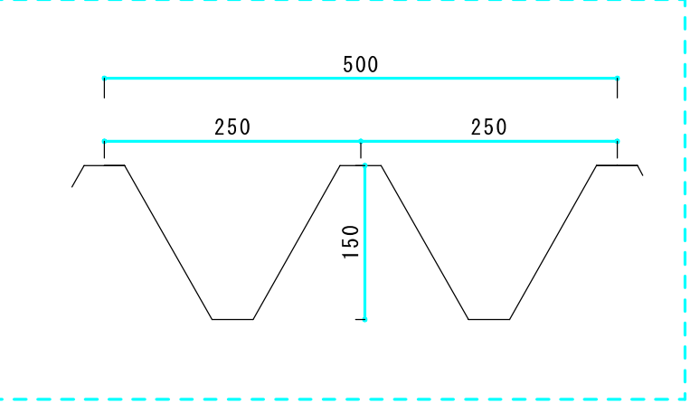
ルーフデッキH150折板
