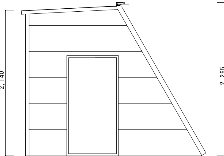
C矢視
