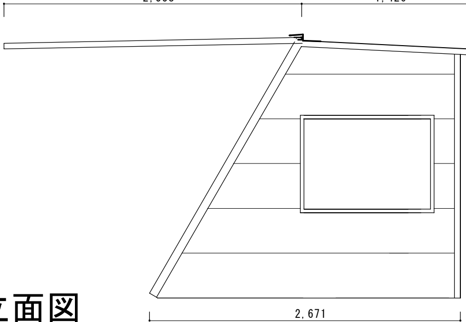
D矢視
